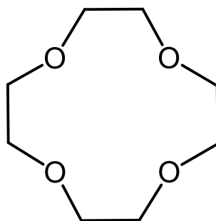
12-クラウン-4 (12員環, 酸素4個)
